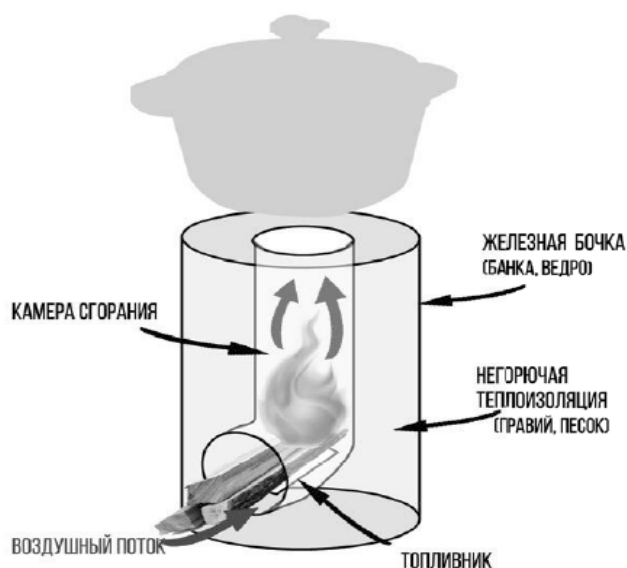
Рис. 9. Ракетная печь из двух консервных банок (водосточной трубы) различного диаметра
