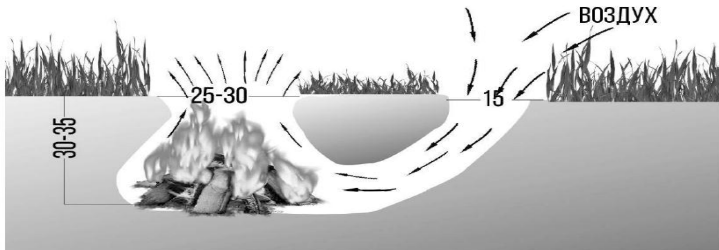
Рис. 8. Костер разведчика бездымный
