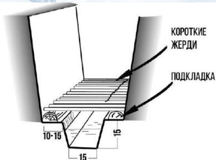
Рис. 3. Перекрытая водоотводная канава на дне траншеи
