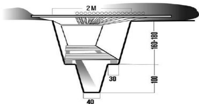
Рис. 4. Отхожее место в траншее, оборудованное поддоном
