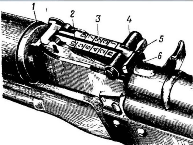
Рис. 15. Прицел автомата и способ его установки
