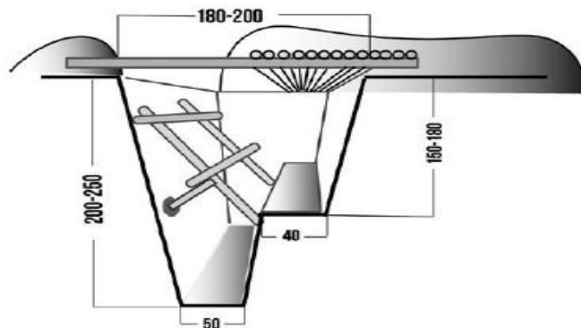
Рис. 5. Отхожее место в траншее оборудованное жердями
